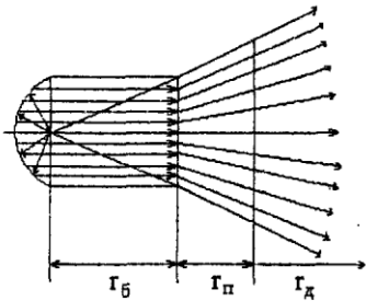
Рис. 3. Межі зон при спрямованому випромінюванні
